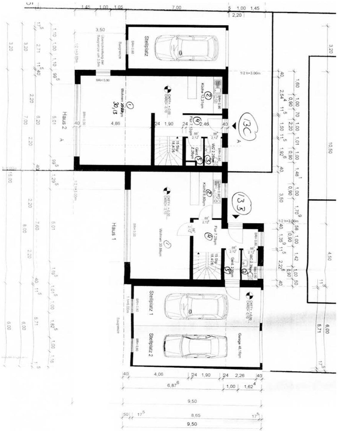
Grundriss Erdgeschoss
