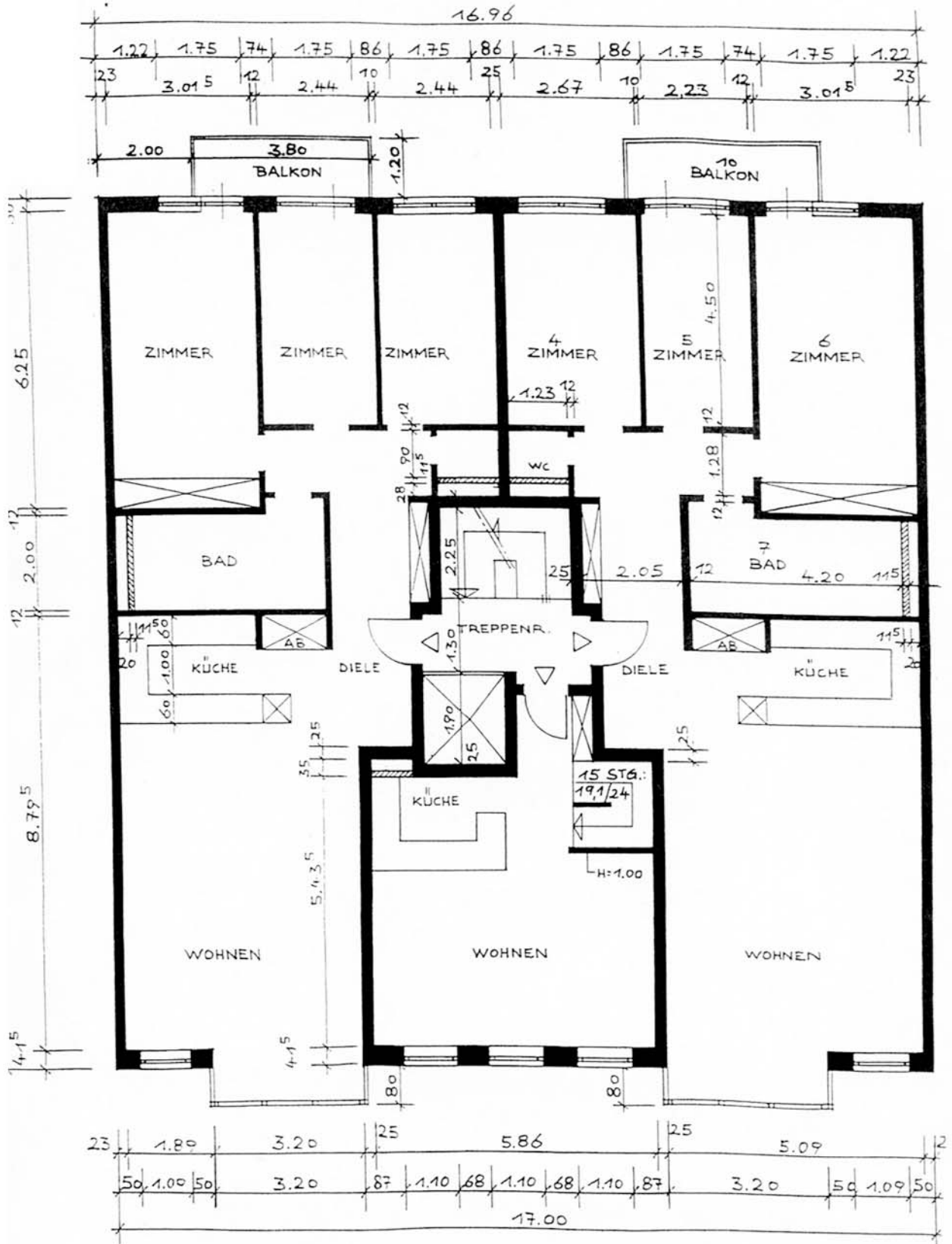
3. OBERGESCHOSS
